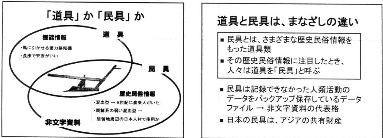
図2 道具と民具
