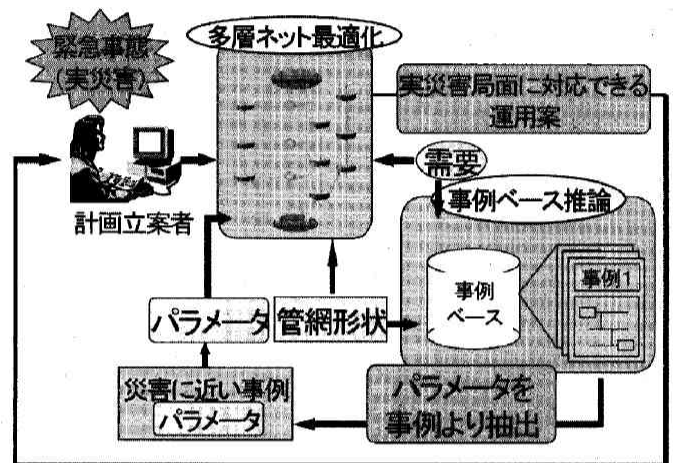
図2 「事例ベース推論+多層ネット最適化」による緊急時水運用管理システム
