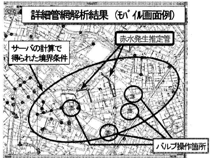
図7 平常時における保守作業支援の事例
