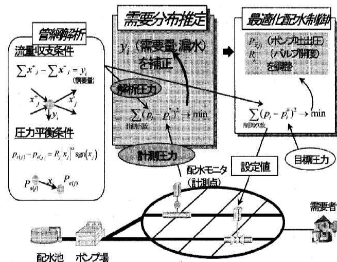
図3 緊急時配水制御システム
