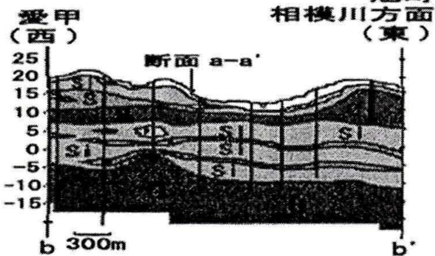
断面 2b-b'
