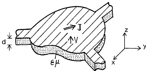
Fig.1 Planar Circuit.
